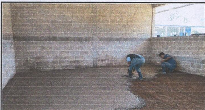
Foto 4: Vista desde el interior de las aulas al momento de realizar la fundición de la torta de concreto.
